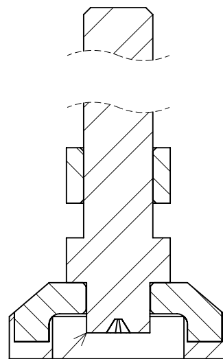
断面図 A-A
