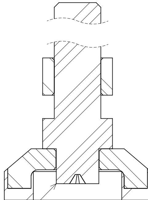
断面図 A-A
