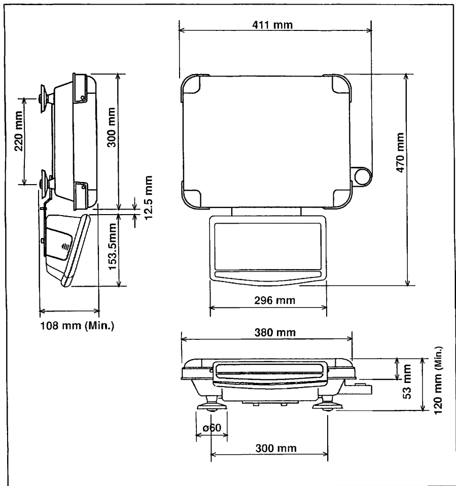
图A-1. 外形尺寸图
