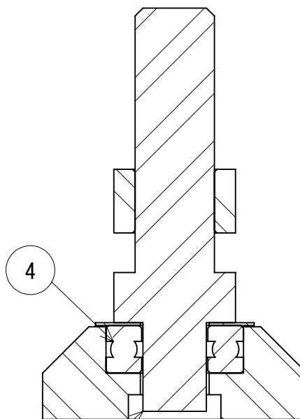
断面図 A-A
