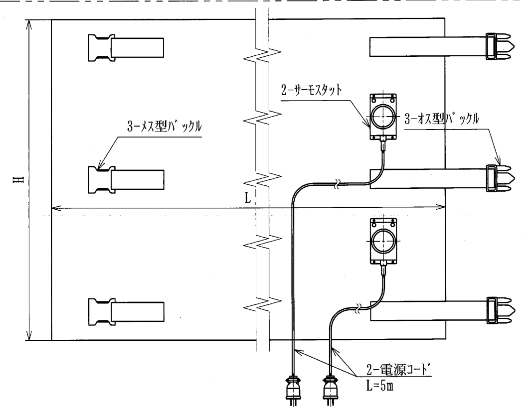
△ B詳細図 (型式:HTJ-HP2D ハックル:3ヶ サーモスタット・電源コード:2ヶ)
