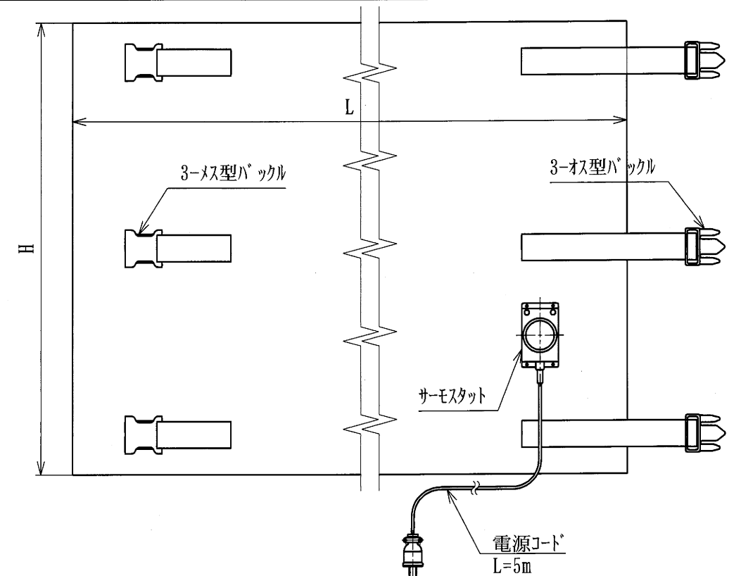
△ A詳細図 (型式:HTJ-HHD ハックル:3ヶ)
