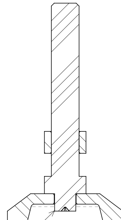
断面図 A-A
