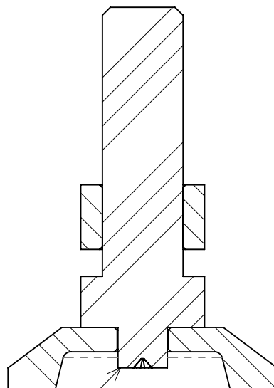
断面図 A-A
