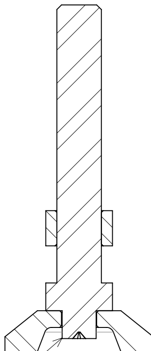
断面図 A-A
