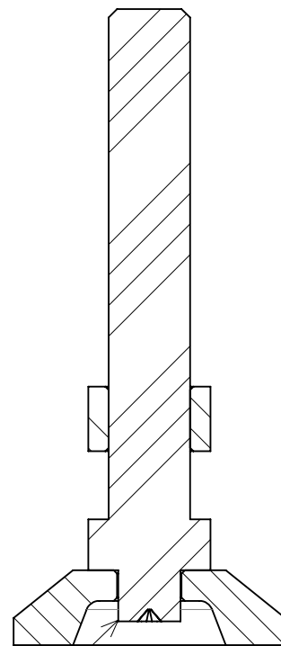
カシメ 断面図 A-A
