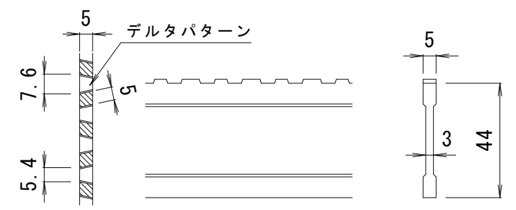
D I - 4 4 バー形状詳細 S = 1 : 2
