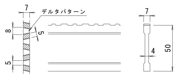
DI-50 バー形状詳細 S=1:2
