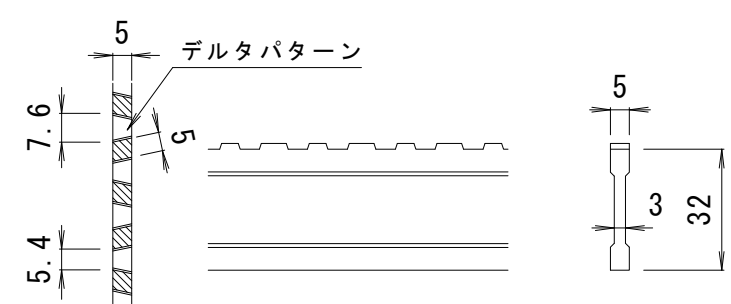
DI-32 バー形状詳細 S=1:2
