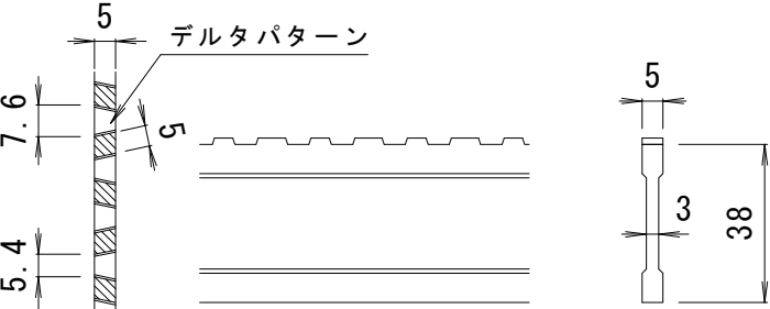
D I - 3 8 バー形状詳細 S = 1 : 2
