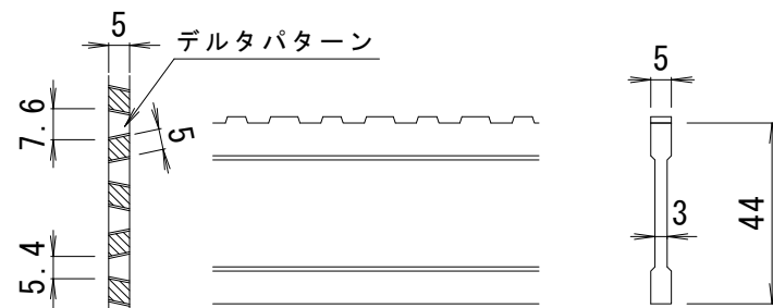
DI-44 バー形状詳細 S=1:2
