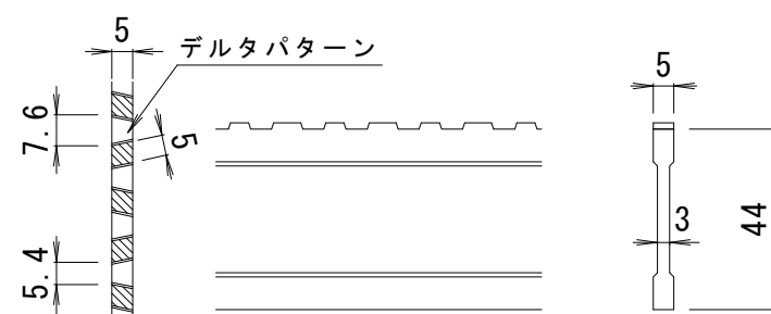
D I - 4 4 バー形状詳細 S = 1 : 2
