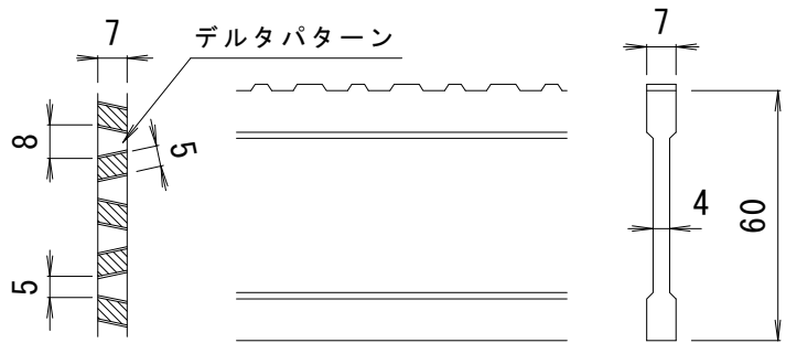
D I - 6 0 バー形状詳細 S = 1 : 2
