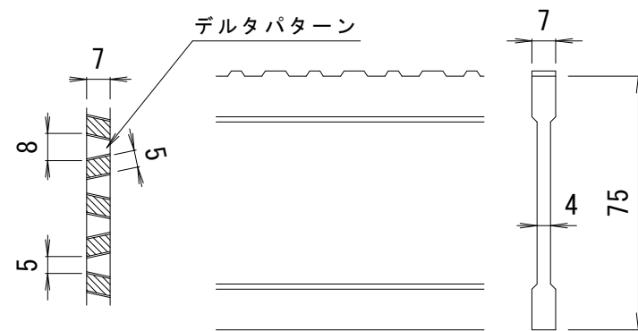
D I - 7 5 バー形状詳細 S = 1 : 2
