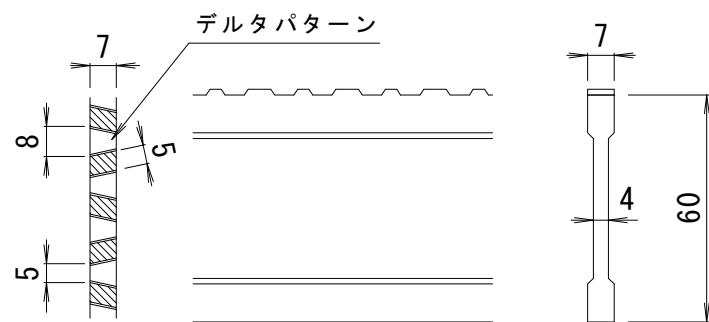
D I - 6 0 バー形状詳細 S = 1 : 2
