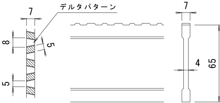
D I - 6 5 バー形状詳細 S = 1 : 2
