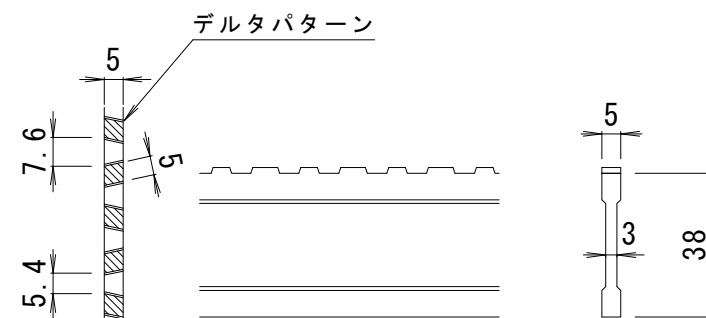
DI - 38 バー形状詳細 S = 1 : 2
