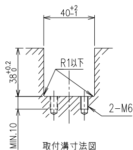
取付溝寸法図
