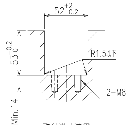
取付溝寸法図
