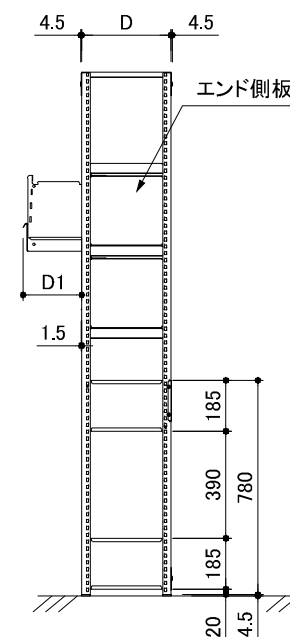
支柱形状
