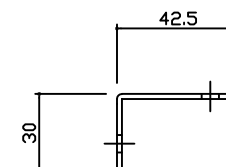
支柱形状
