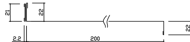
棚板詳細図
