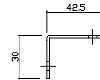
支柱形状
