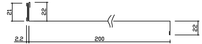
棚板詳細図
