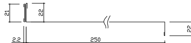
棚板詳細図
