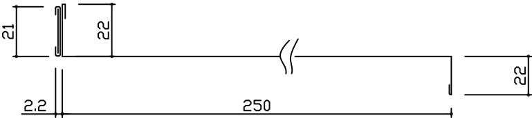
棚板詳細図
