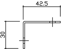
支柱形状
