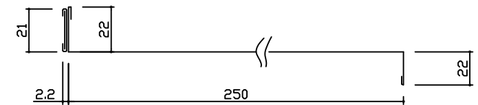
棚板詳細図
