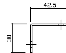
支柱形状
