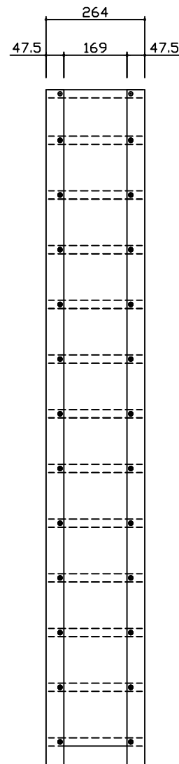
棚板詳細図
