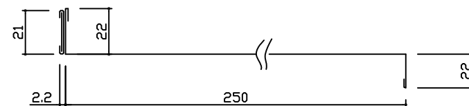
棚板詳細図
