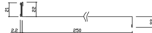
棚板詳細図
