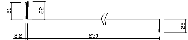
棚板詳細図
