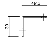
支柱形状
