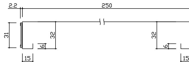
棚板詳細図
