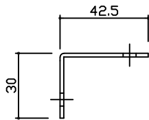
支柱形状
