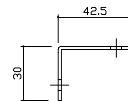
支柱形状
