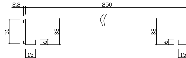
棚板詳細図
