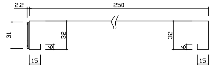
棚板詳細図
