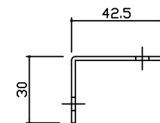
支柱形状
