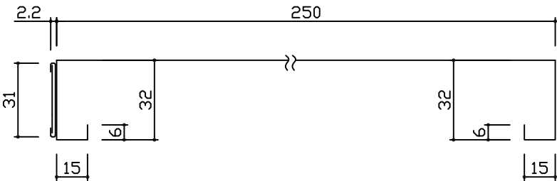
棚板詳細図
