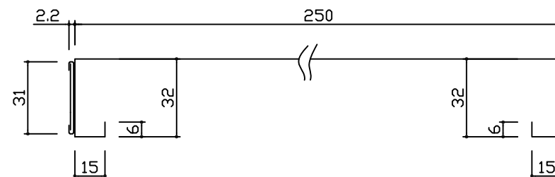
棚板詳細図
