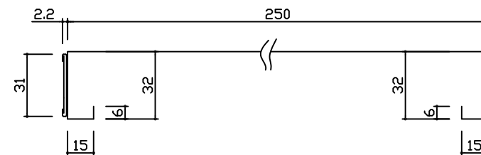
棚板詳細図
