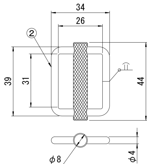
本体金具詳細図
