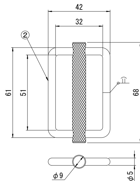
本体金具詳細図
