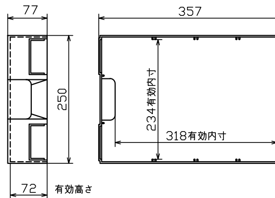
引出詳細図
