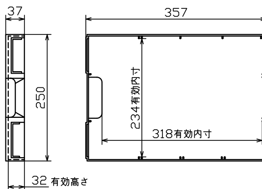
引出詳細図
