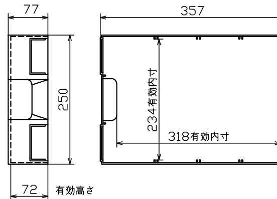
引出詳細図
