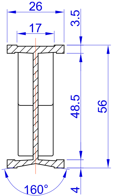
A-A' 断面
