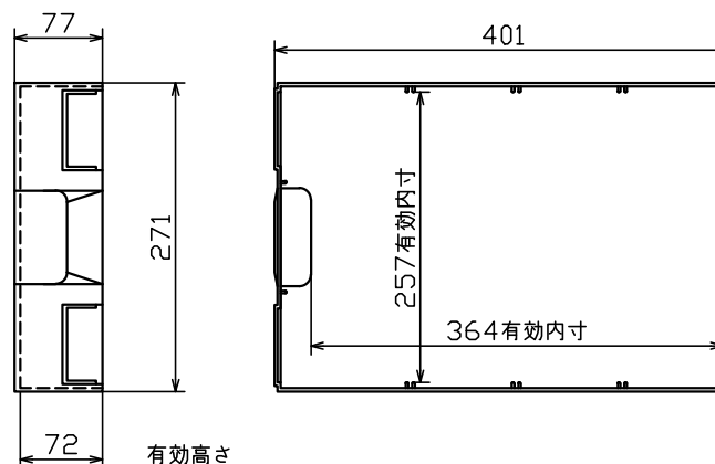
引出詳細図
