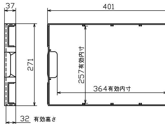
引出詳細図
