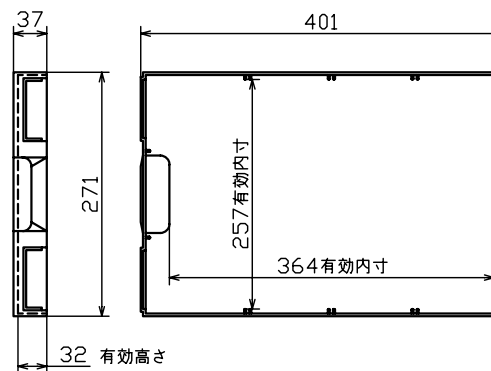
引出詳細図
