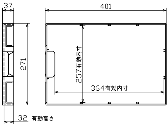
引出詳細図
